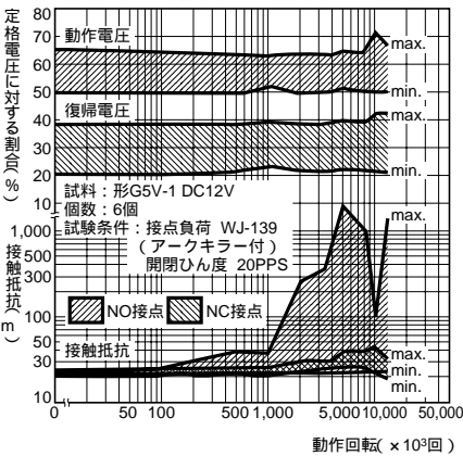
ダイヤルパルス試験 *1
