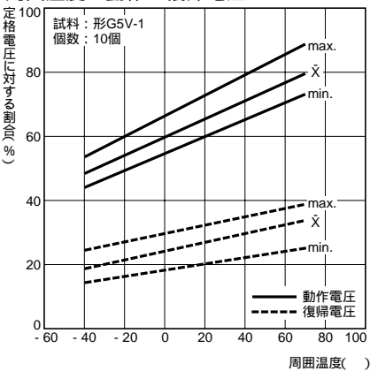
周囲温度と動作・復帰電圧
